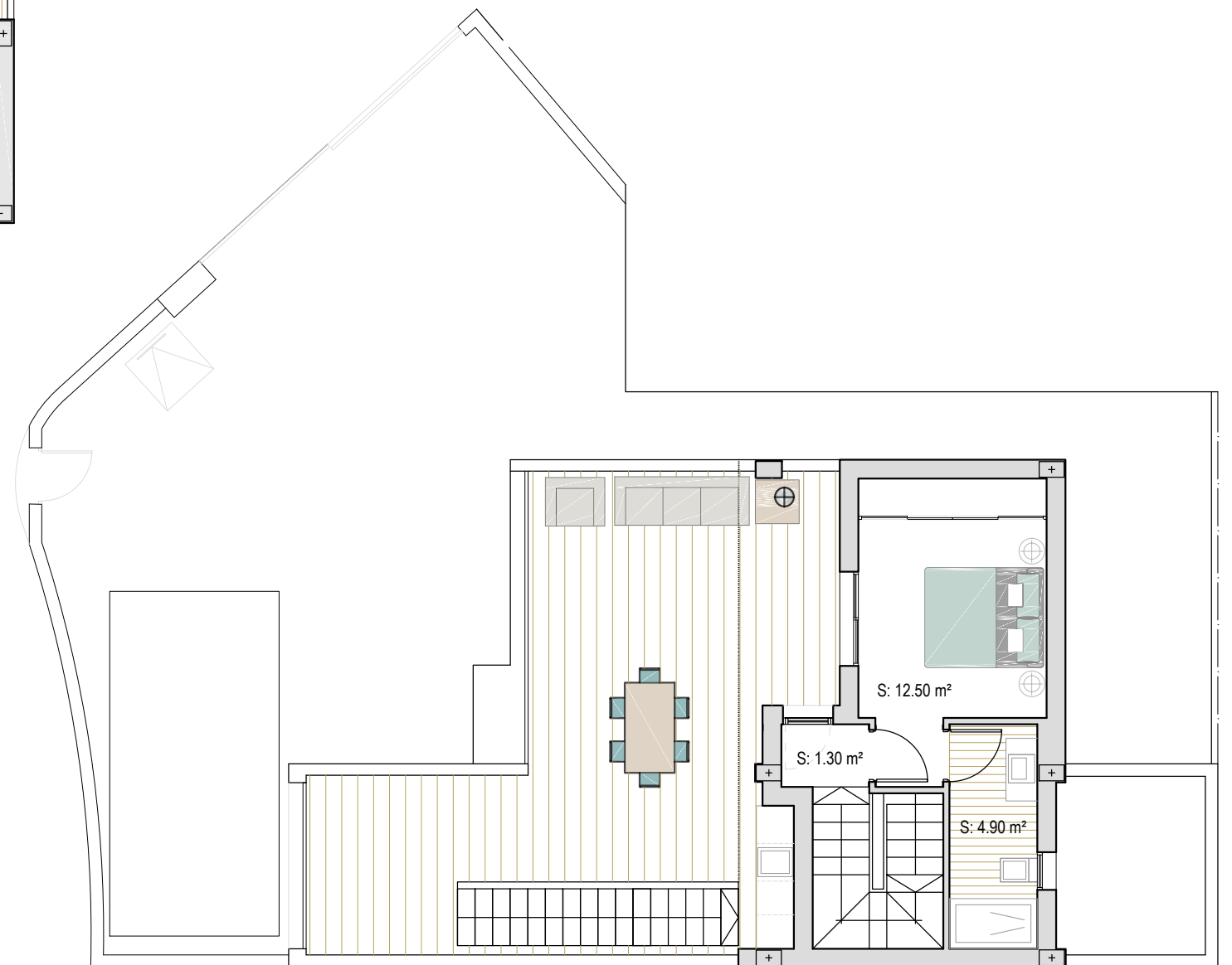
Planta primera
