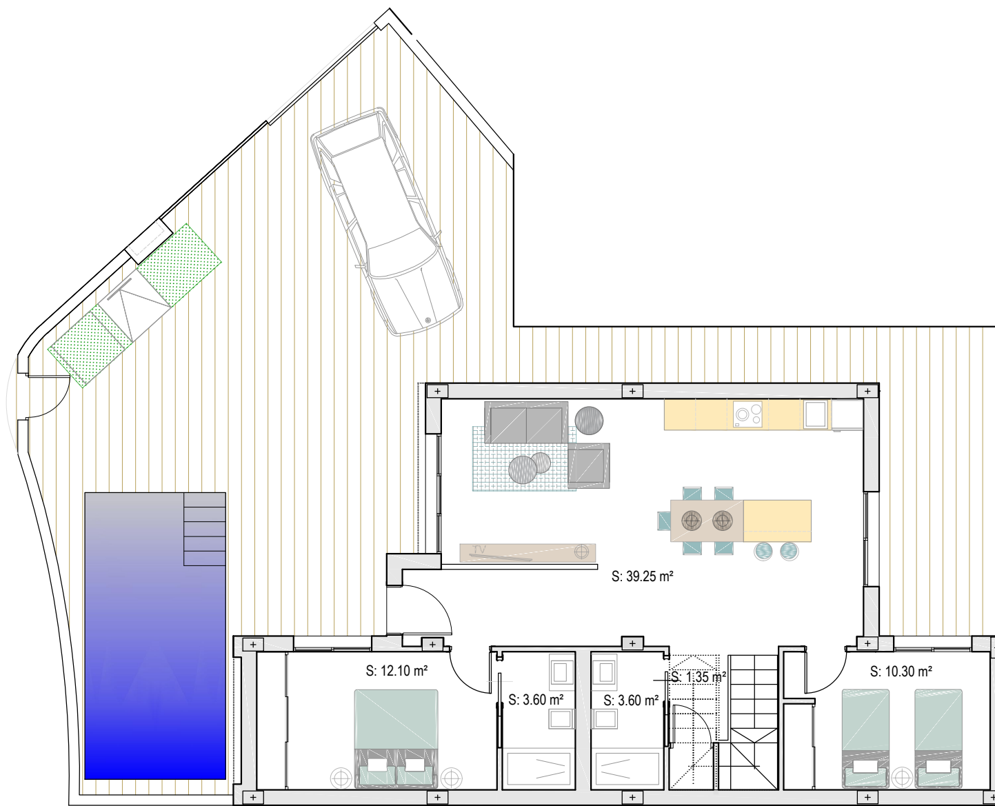
Planta baja
